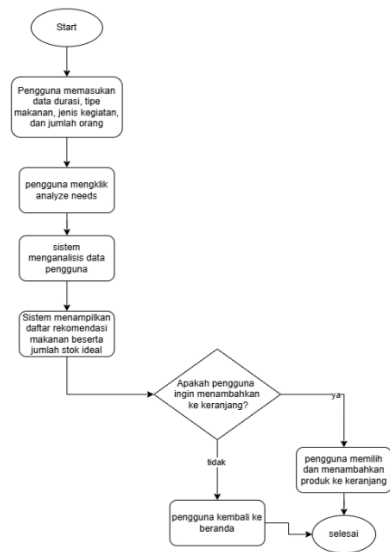
Gambar 2. flowchart fitur analisis kebutuhan stok
