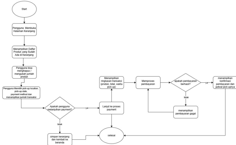
Gambar 5. flowchart fitur transaksi
